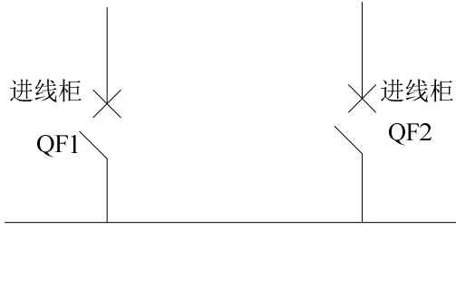
图 1.18 (b) 两进线无母联
