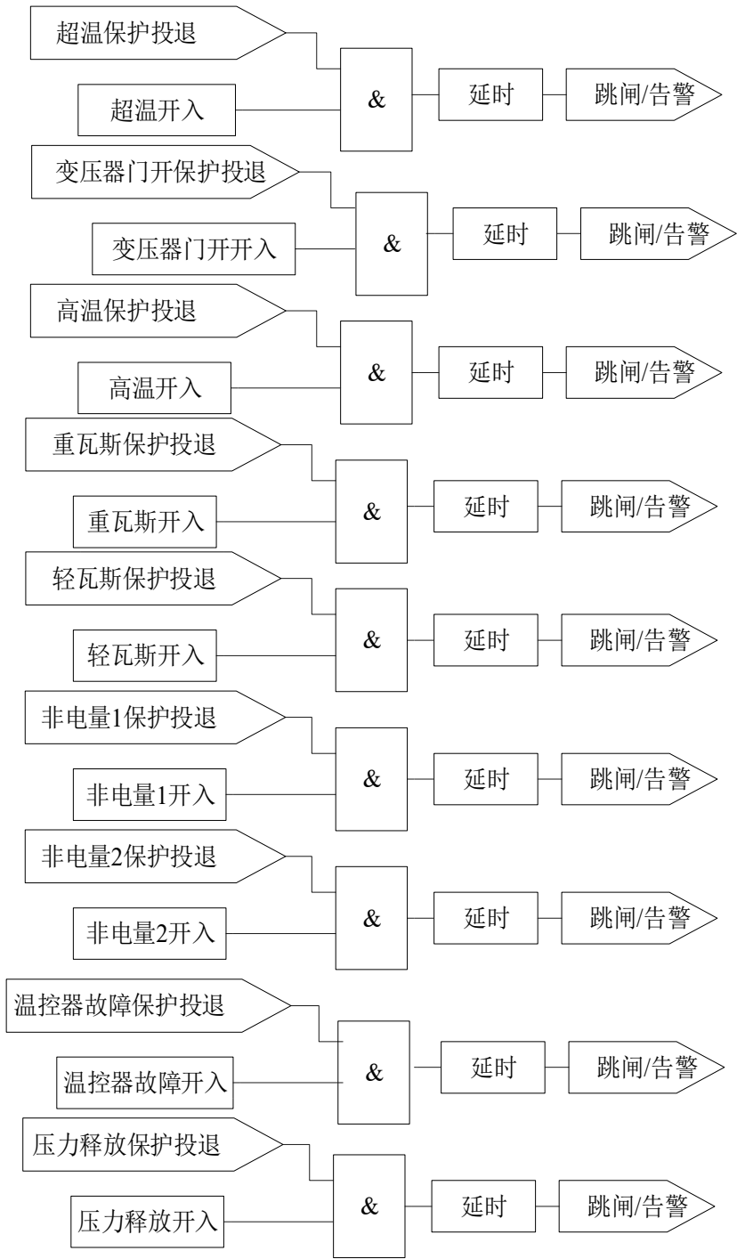
图 1.13 非电量保护逻辑
