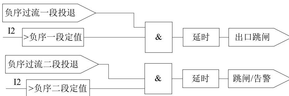
图 1.11 两段式负序过流保护逻辑
