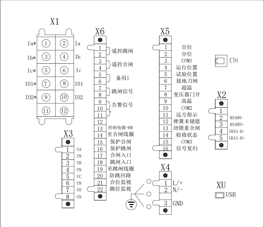
图 1.19 AM4-I 电气接线图
