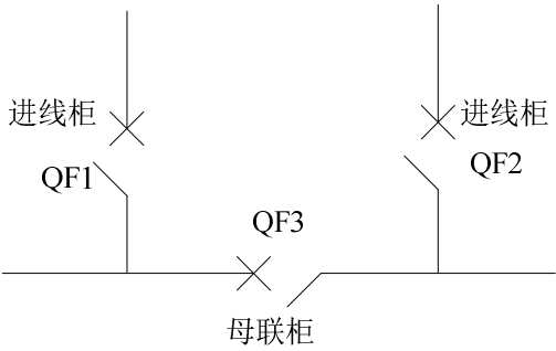
图 1.18 (a) 两进线-母联
