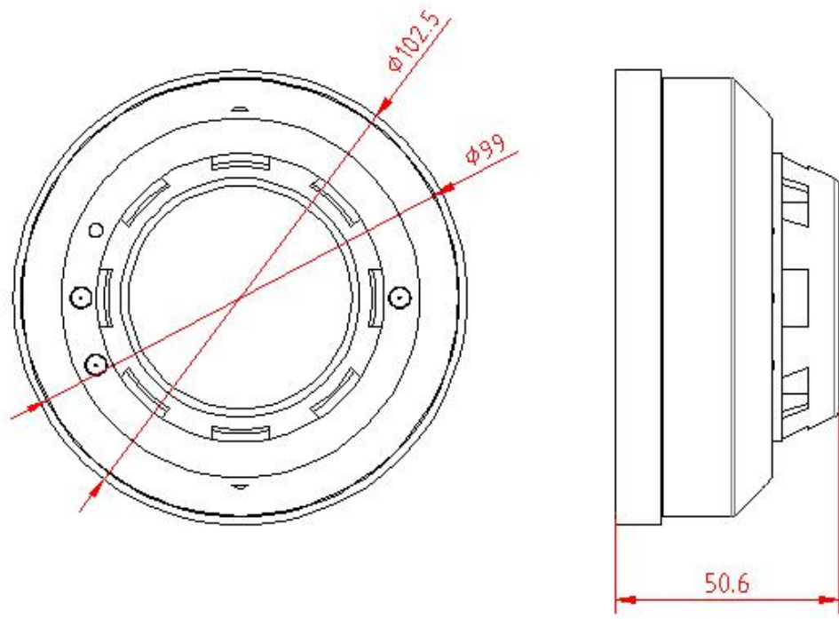
图1 外形尺寸图
