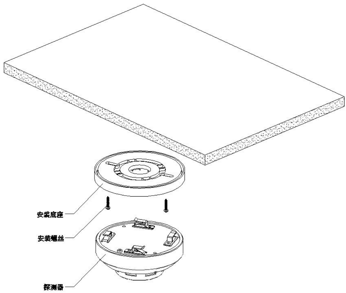
图2 安装示意图
